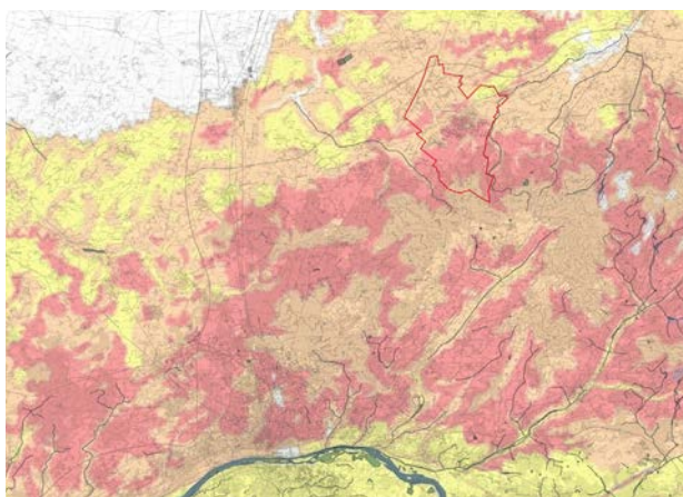
Aléa retrait/gonflement des argiles
