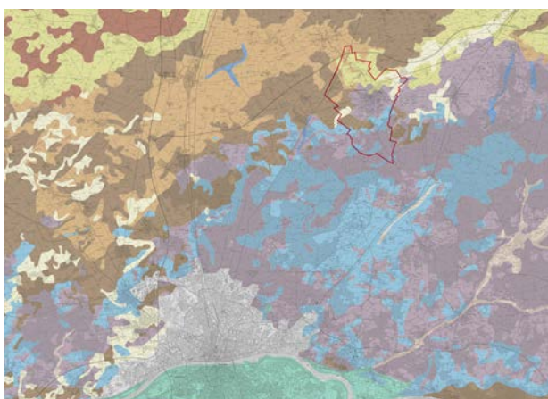
Qualité des sols
